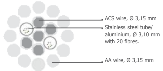
OPGW AS/AA 39/94 AST 2 x 20F:
